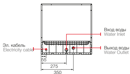
Вид сзади / Back of dishwasher
