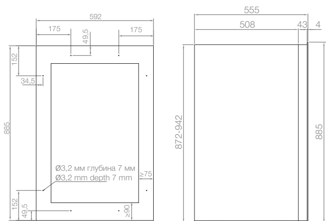
Размеры панели / Panel dimensions
